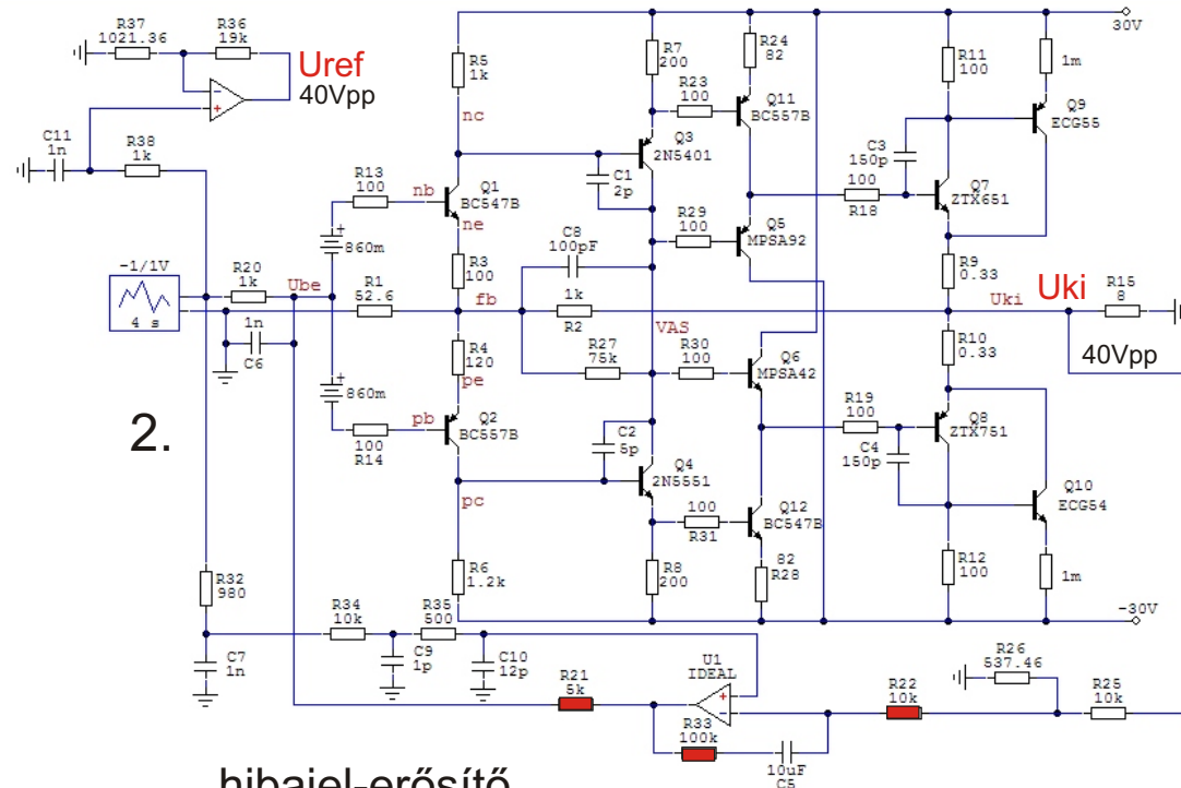
hibajel-erősítő
