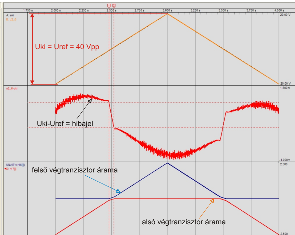
DC szervó
