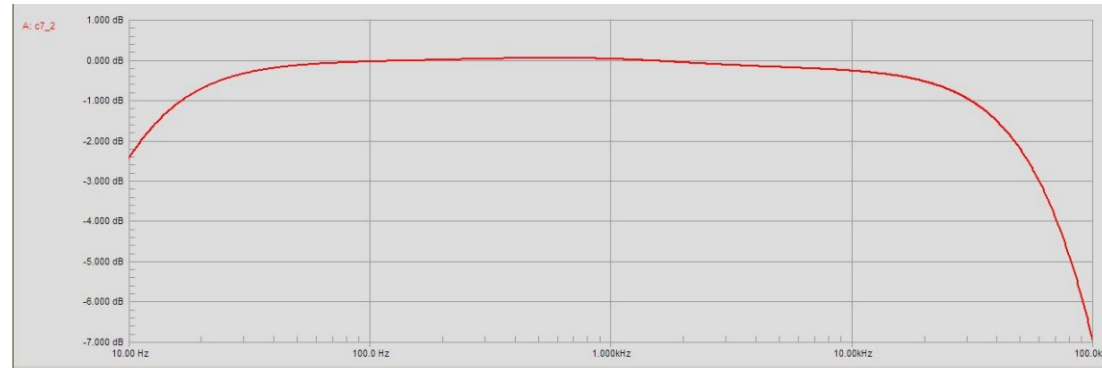
lineáris 10Hz - 30kHz (-1 dB)
