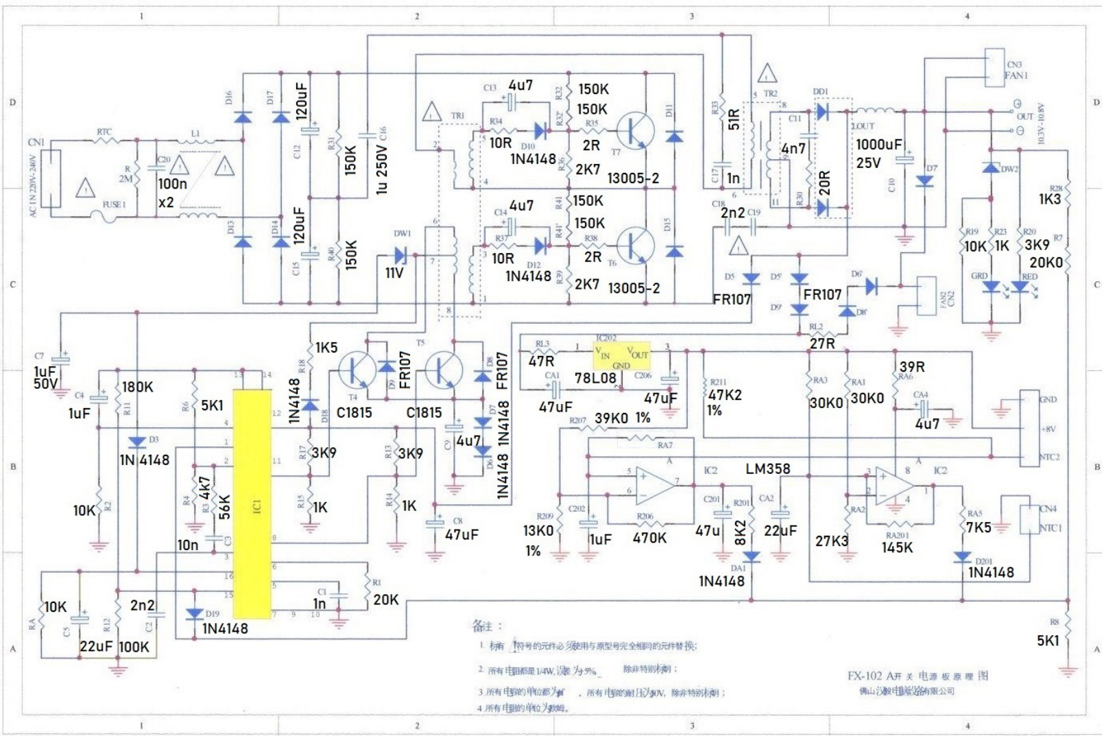
FX -101 FX-102 A PCB90829F1 SCH:
