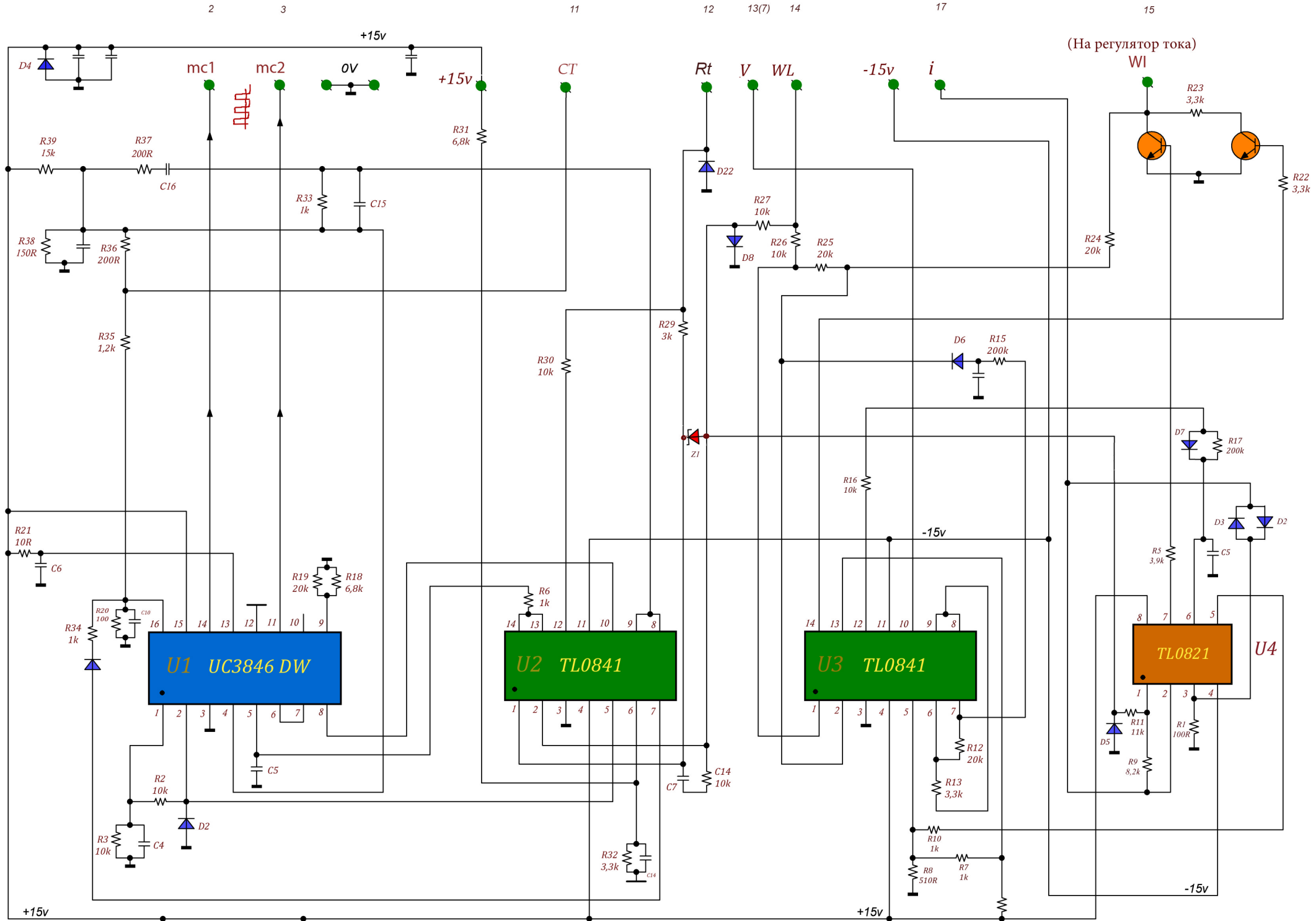
Микро СВИ-205 (схема управления)
