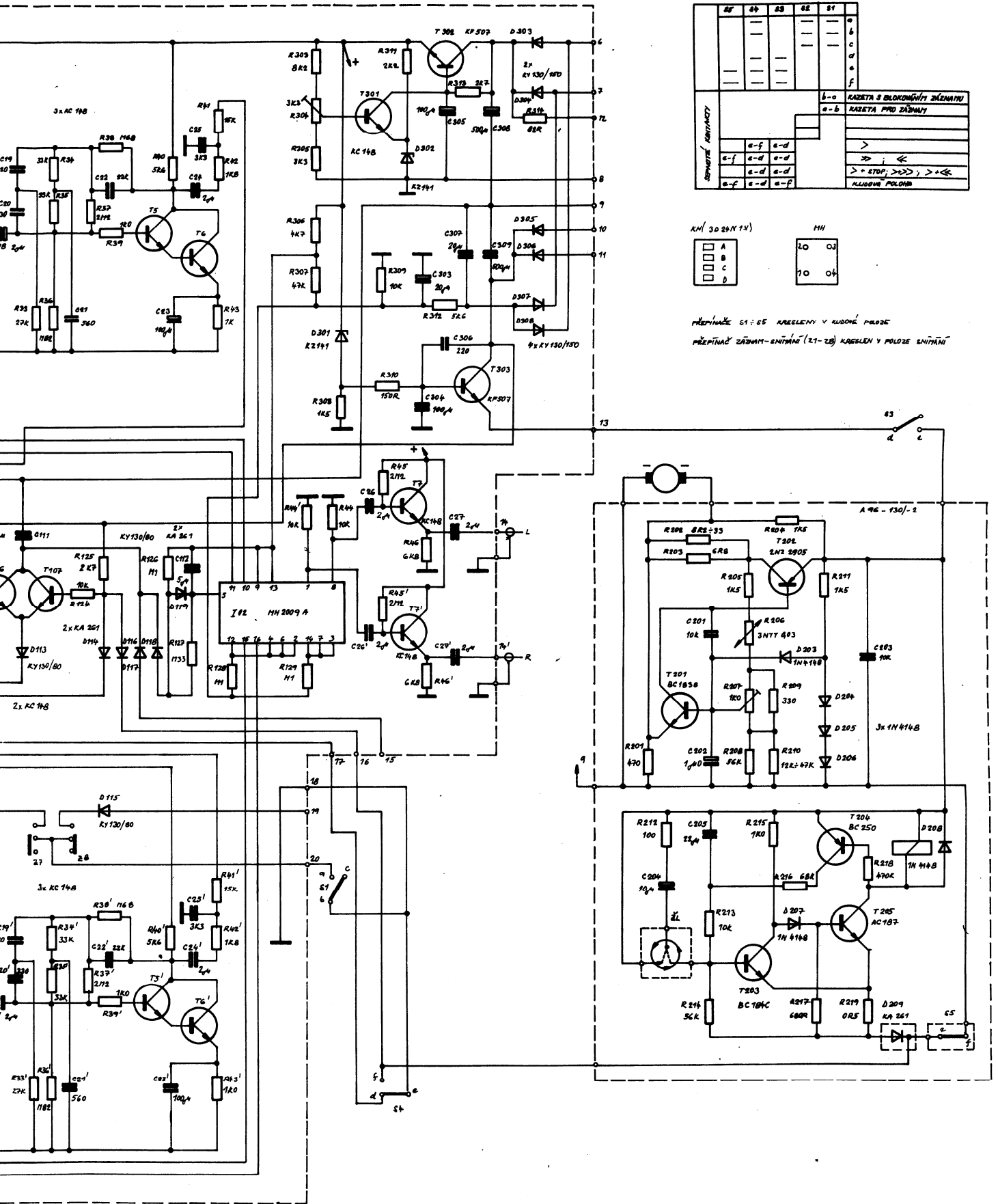
ojení magnetofonové jednotky
