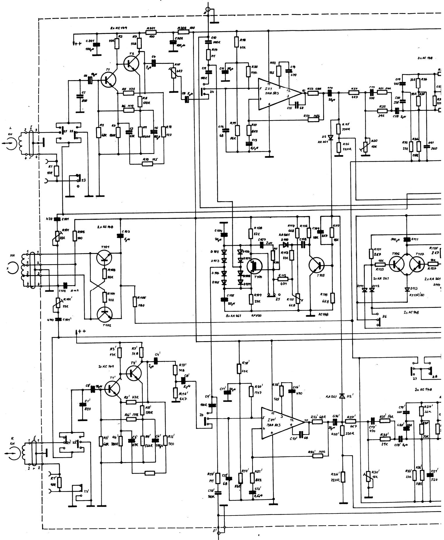
Obr. 5. Schéma zapojení magne
