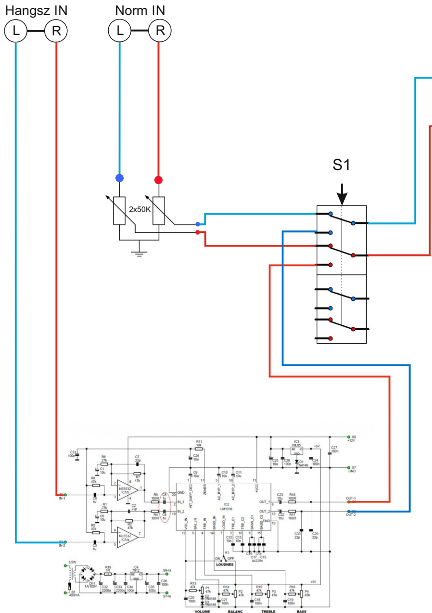
Előerősítő + szint és hangszínszabályzó LM1036-al
