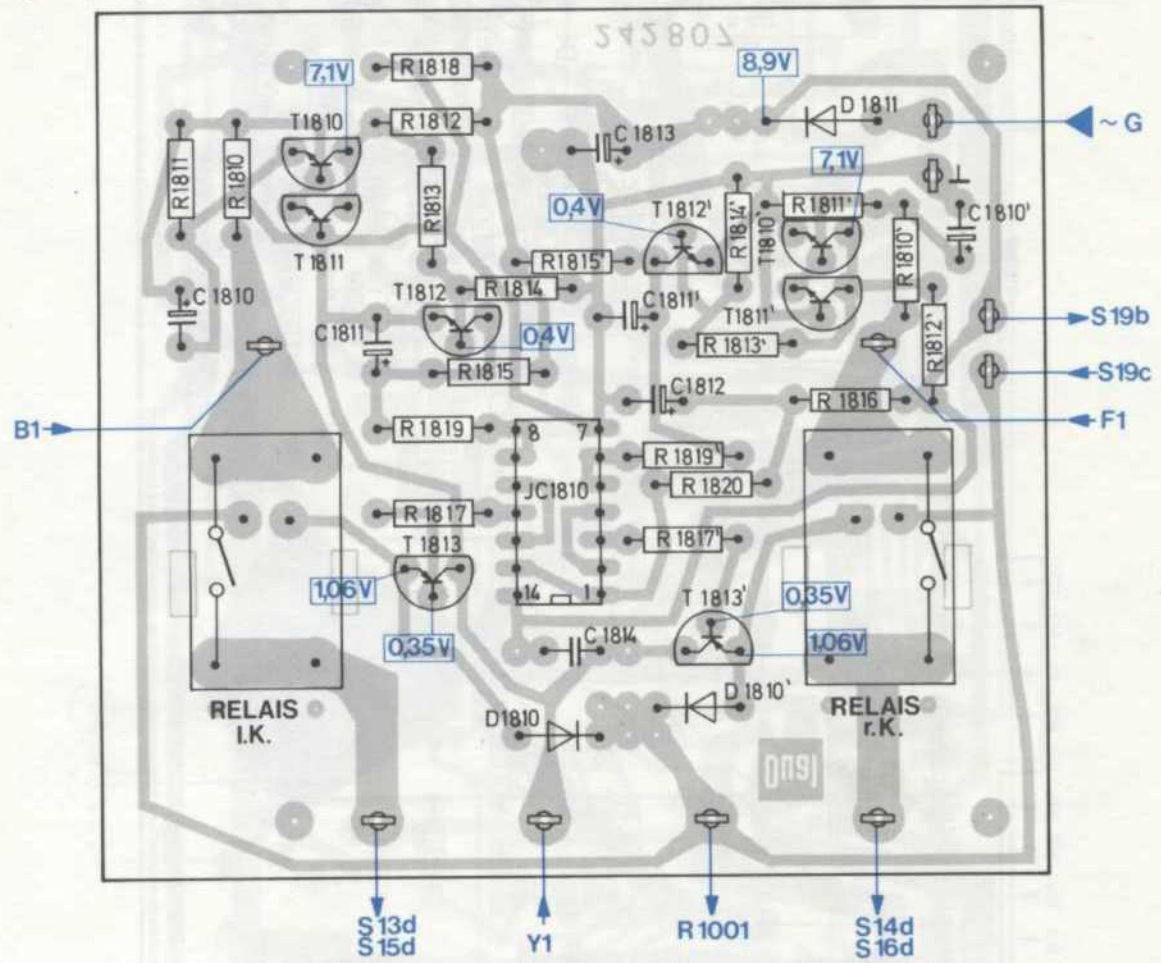
Fig. 17 Lautsprecherschutzplatte 243 519 (Bestückungsseite)
