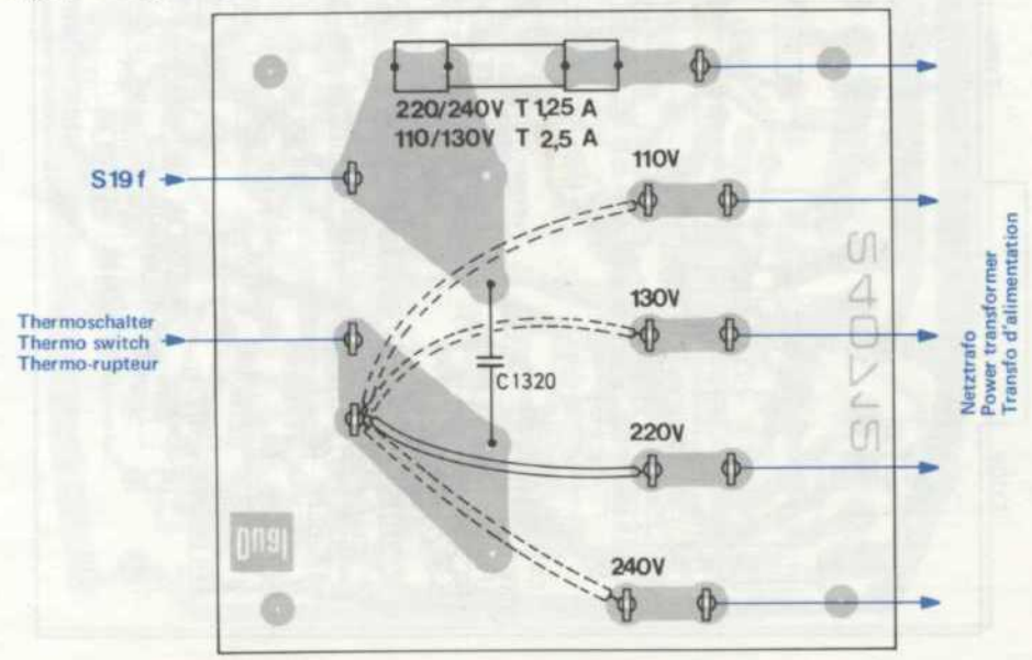
Fig. 18 Netzplatte 240 711 (Bestückungsseite)
