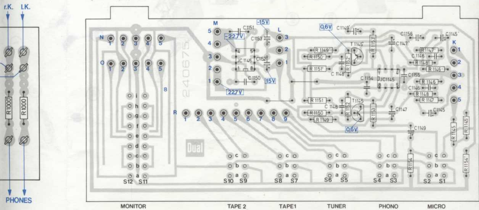
Fig. 21 Eingangswahlschalter 243 724 (Leiterseite)
