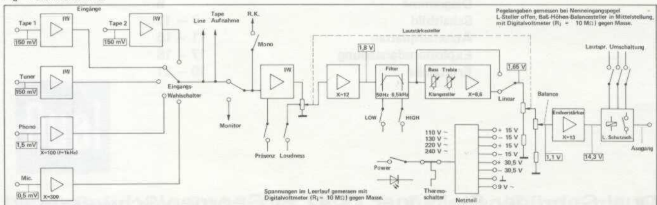
Fig. 1 Blockschaltbild
