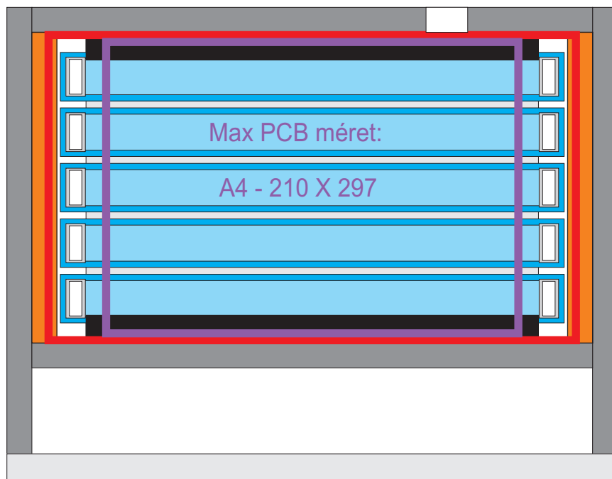
Felülről nézve
