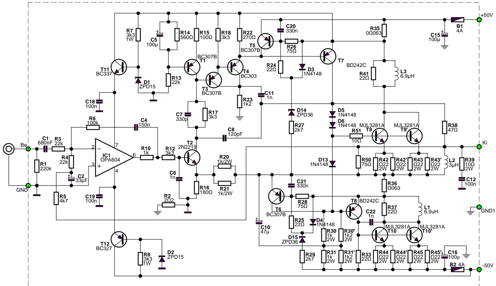
QUAD-405 R.Ludvig féle módosítása (ALKOTÓ-s átrajzolatban)
