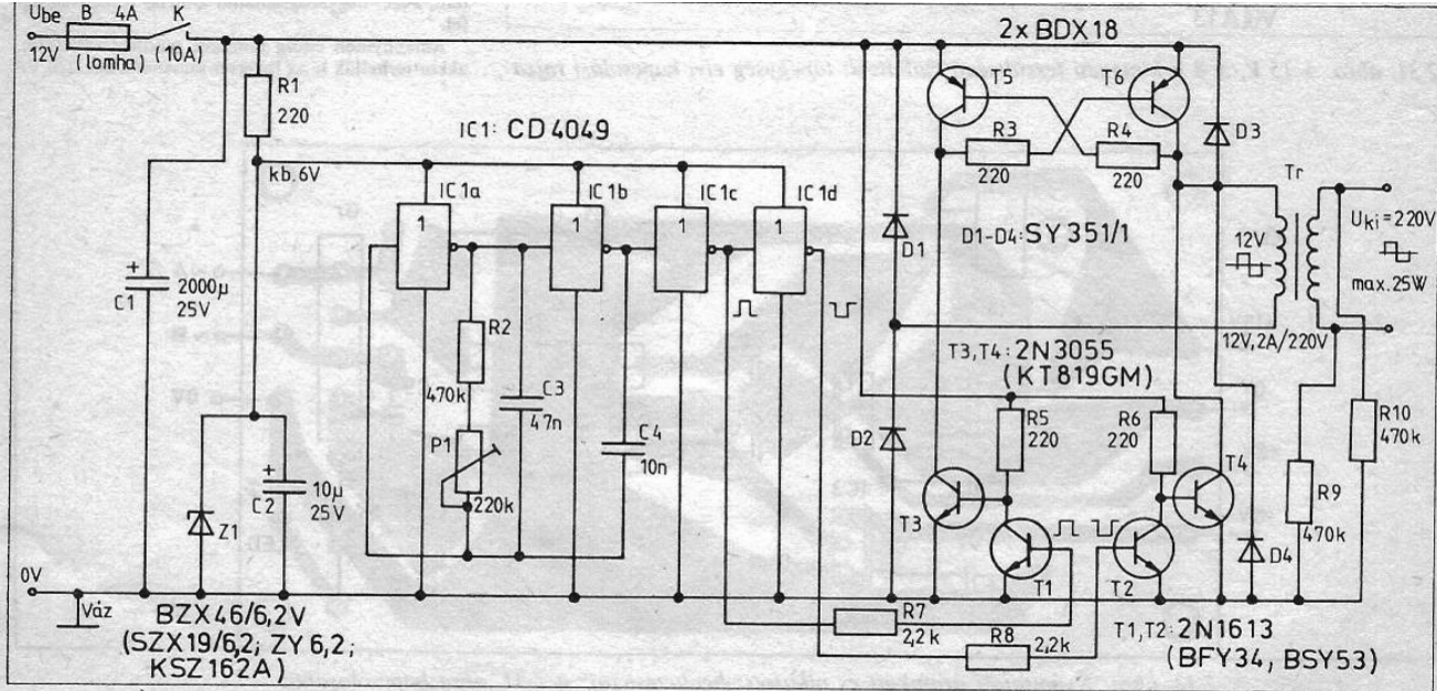
3.2. ábra. 12 V/220 V, 50 Hz, max. 25 W terhelhetosegu, szabályozatlan kimeneti feszültségű DC-AC inverter
