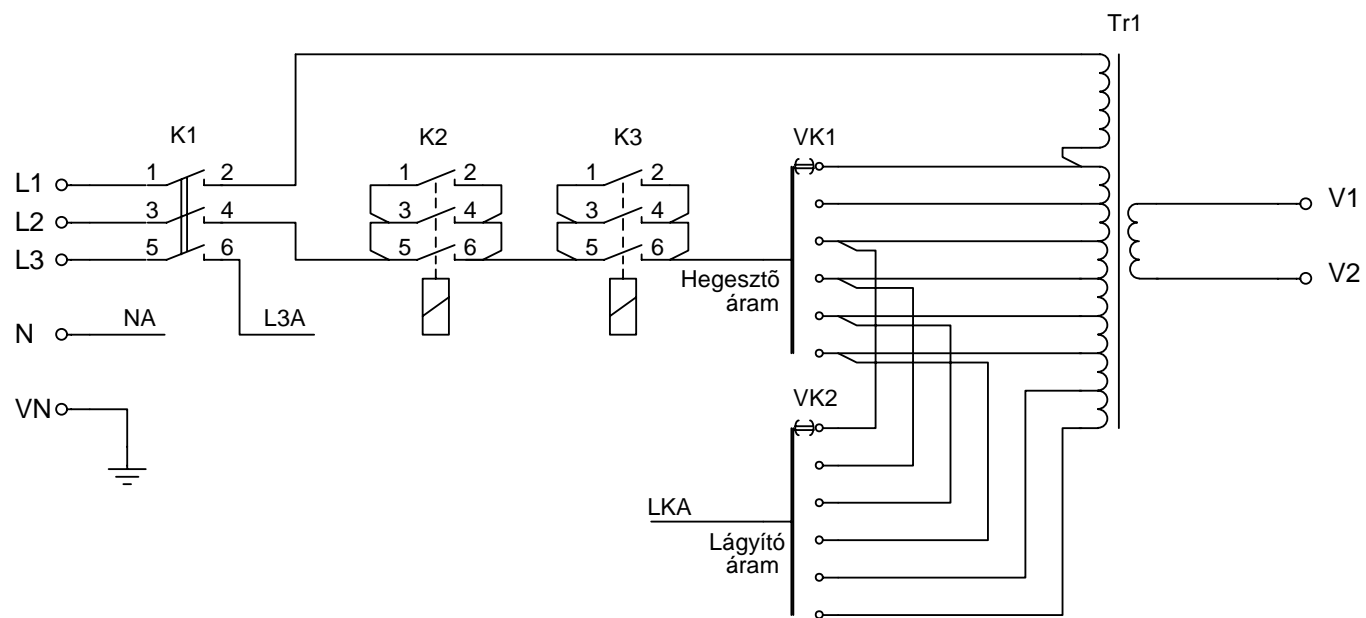
VEB BSG32/40 szállagfűrész lap hegesztő gép főáramkör
