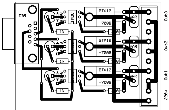
3 Sorties Sur Triacs v2.2 - Copyright (C) 2009 Dani Imre (valve)
