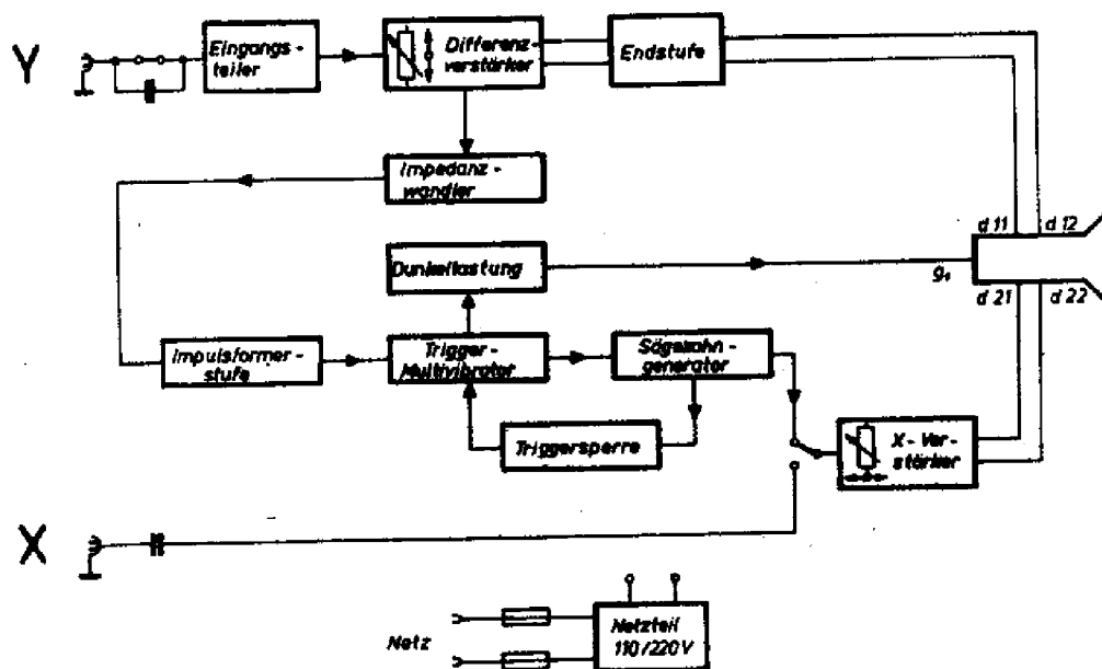
Blockschaltbild EO 201
