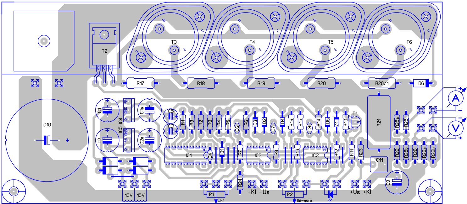
ALKATRESZ OLDAL
