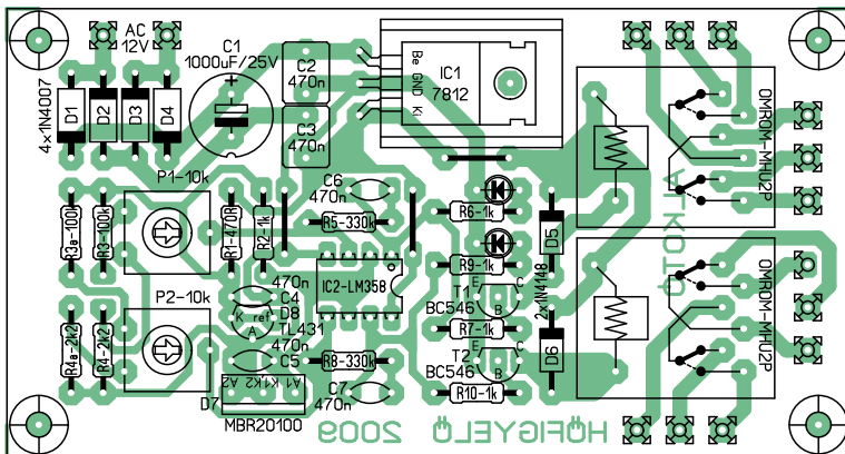
ALKATRESZ OLDAL
