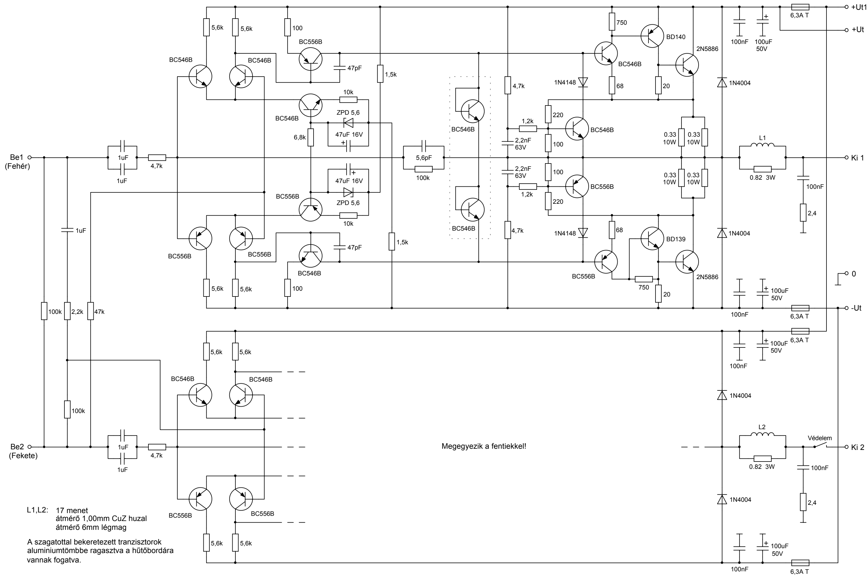
REFLEX RX-500 Végerősítő - erősítő panel (egyik csatorna)
