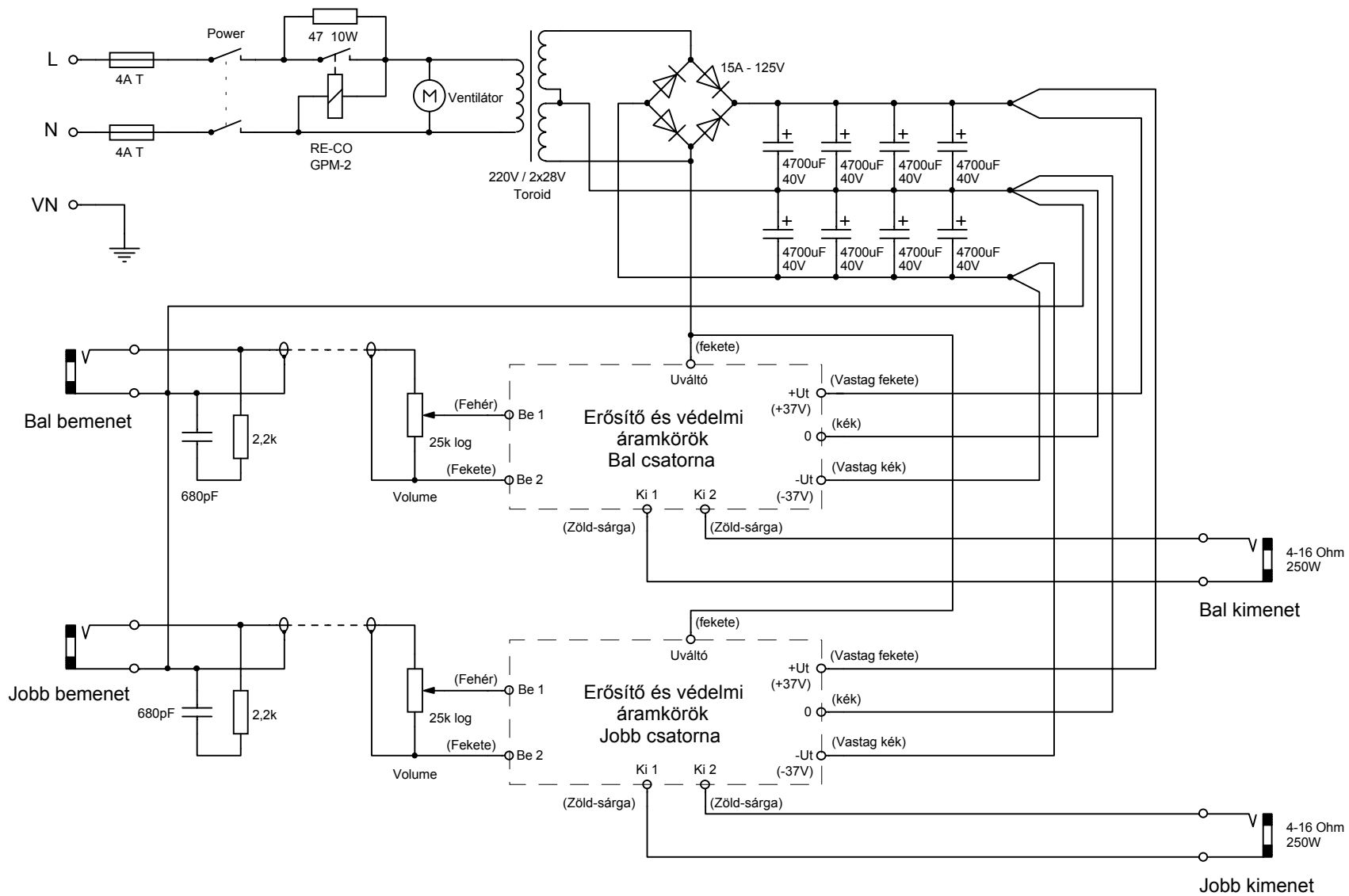
REFLEX RX-500 Végerősítő - Tápegység és az összehuzalozás
