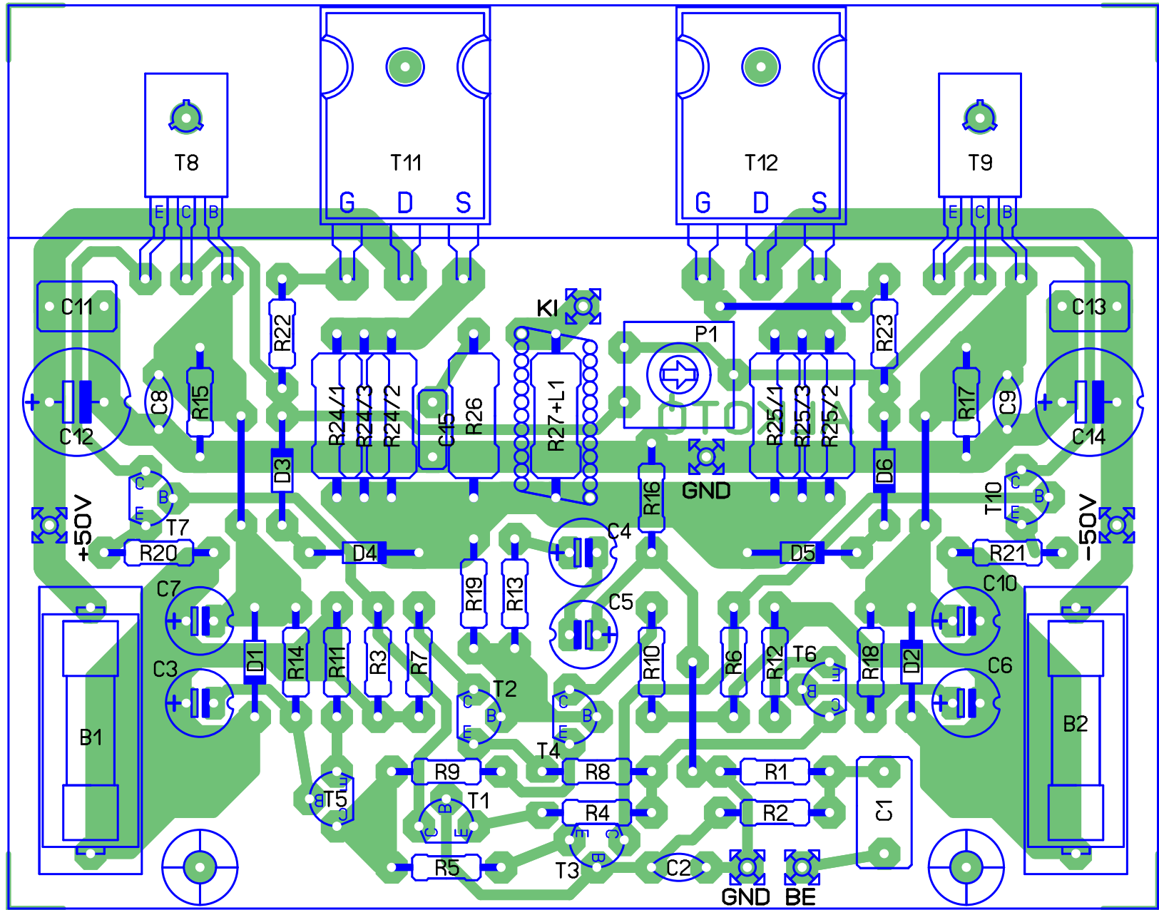
MONACOR PMA 100 panelterv-v1.0 (alkatresz oldal)
