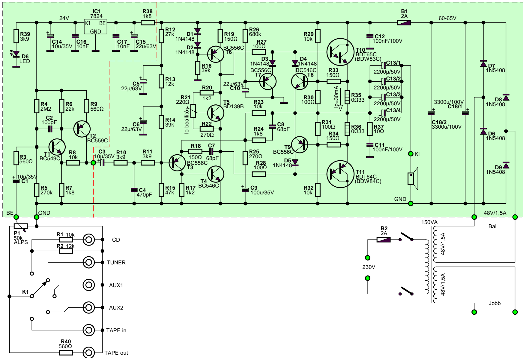
HT A30 végerősítő (Alkotó-s ábrázolata)
