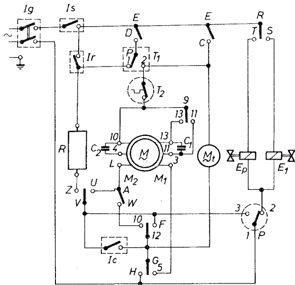
5.25. ábra. HIM 706 típusú automata mosógép kapcsolása
